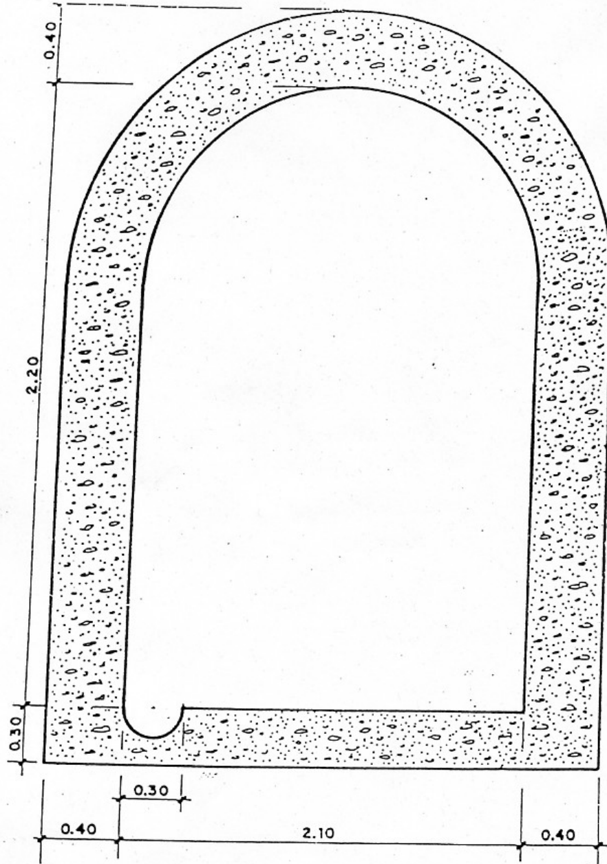
SECCION TIPO DE GALERIA DE SERVICIOS DE BOVEDA-PRINCIPAL
